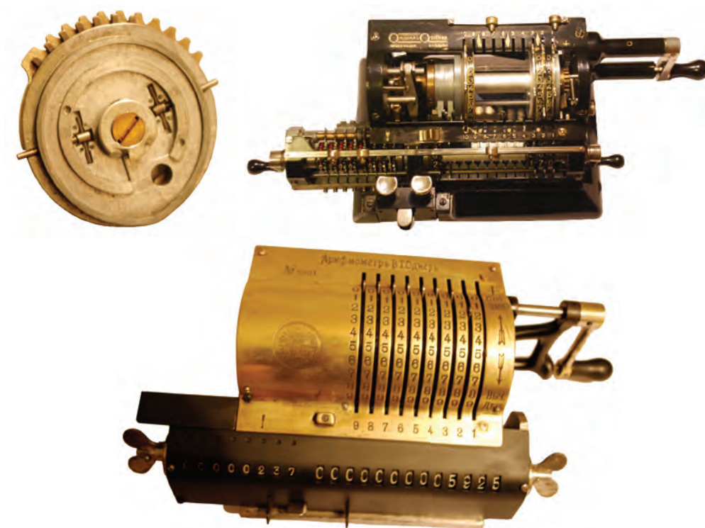
Rysunek 13. Koło z ruchomymi zębami. Demonstracyjny (pocięty) model kalkulatora Original Odhner. Kalkulator Odhnera wyprodukowany w St. Petersburgu (ustawienia po wykonaniu mnożenia 25 \times 237 )
